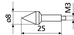
MKe 8
