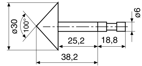
MKe 30
